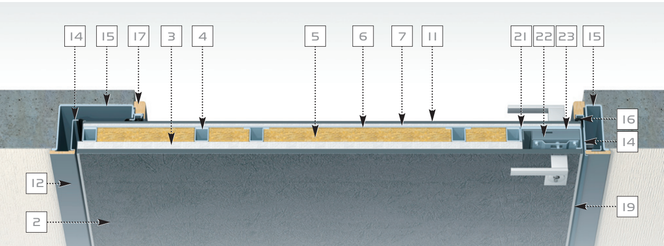
Sezione Orizzontale
